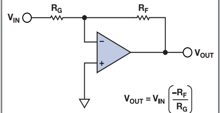
Inverting Op Amp
